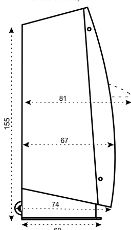
VUE DE COTE AVEC KIT CLAVIER
